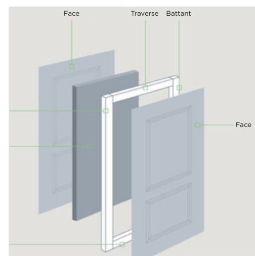
Composition de notre porte à panneaux moulés
